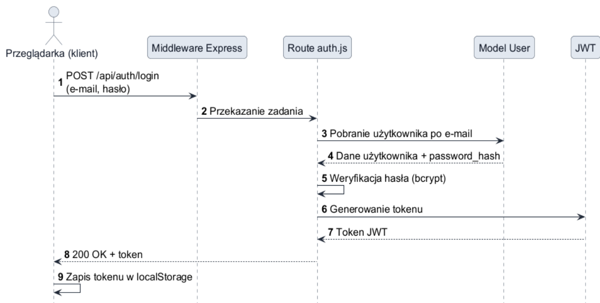
Rys. 3. Diagram sekwencji – logowanie użytkownika
