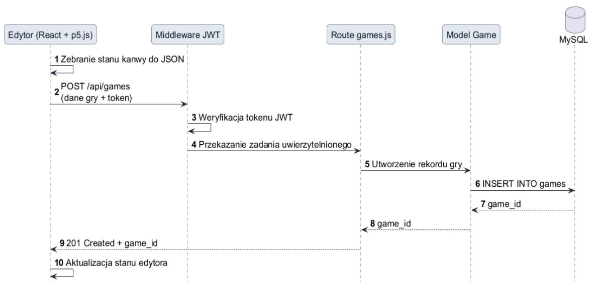
Rys. 4. Diagram sekwencji – zapis gry przez edytor
